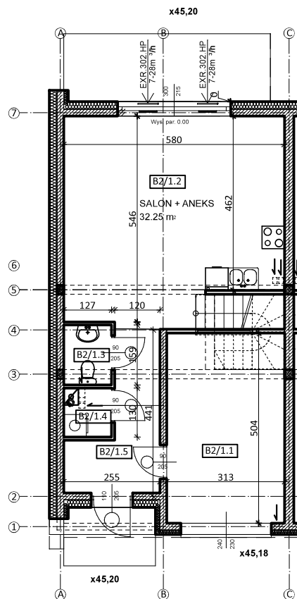
RZUT PARTERU
